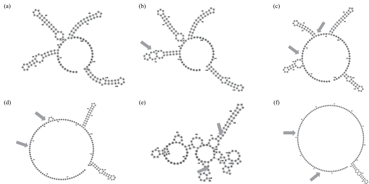
Fig. 7 Secondary structure comparison for sample AE016830.1_3 201 675 (a) Ground truth, (b) RMDfold ( F1 =0.977 2), (c) REDfold ( F1 =0.860 7), (d) sincfold ( F1 =0.676 4), (e) TransUfold ( F1 =0.425 0), (f) Ufold ( F1 =0.392 9).
